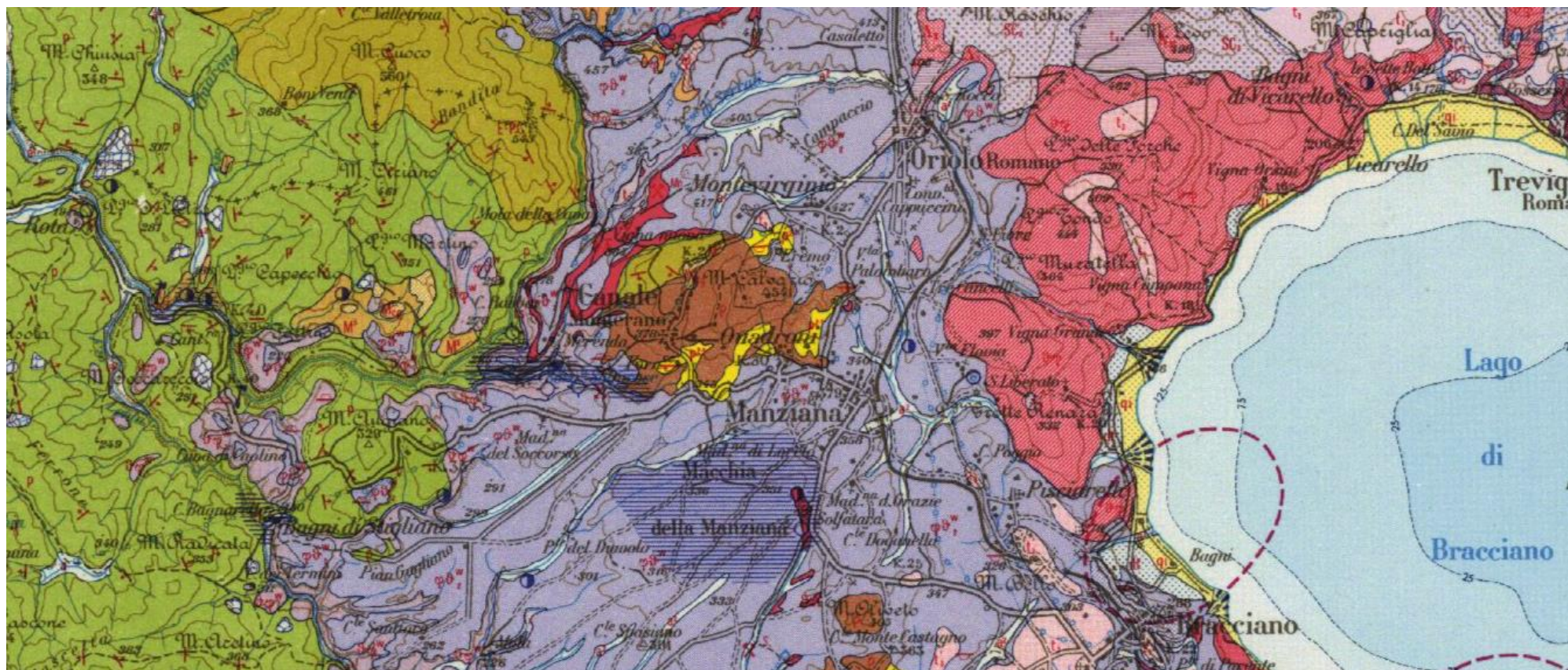
Foglio 143 – Bracciano – Stralcio carta Geologica al 100.000
