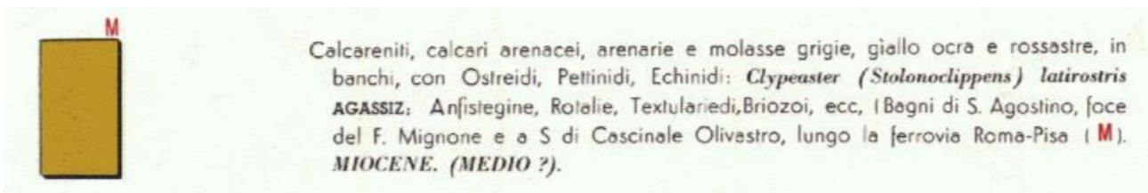
Stralcio carta Geologica scala 1:100.000 – Foglio 142 Civitavecchia
