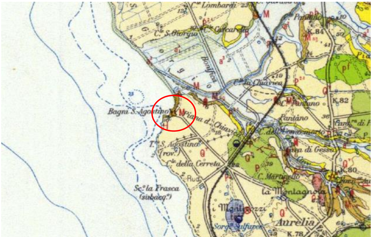
Stralcio carta Geologica scala 1:100.000 – Foglio 142 Civitavecchia
