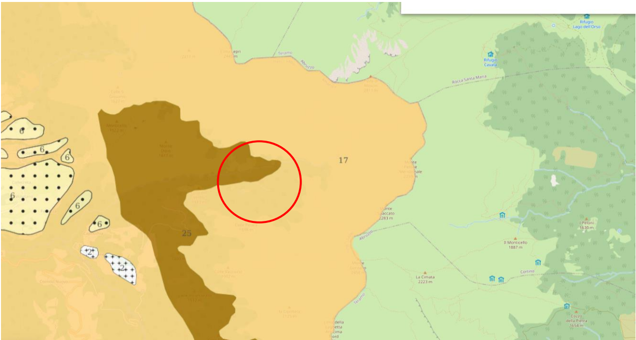
Stralcio Carta Geologica al 25.000 – Geoportale Regione Lazio - Depositi sin-orogenesi di Avanfossa del Miocene superiore; Flysch a componente dominante arenacea o conglomeratico-arenacea .
